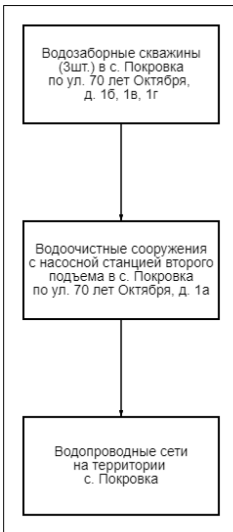
Рисунок 1.1.1 – Структурная схема централизованного водоснабжения СП Покровское
